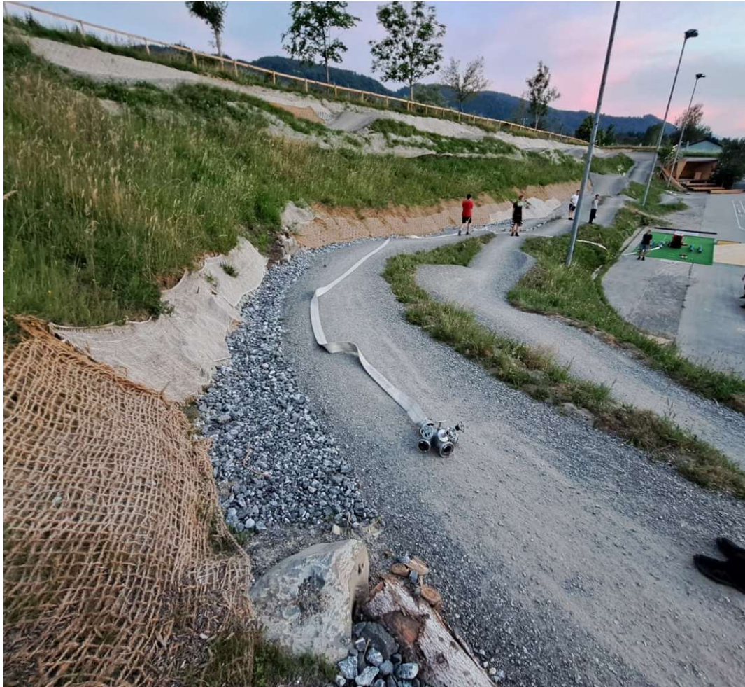
Abb. 4: Zubringerleitung bis Verteiler
